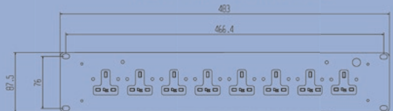
D13-08H 2U 8 WAY HORIZONTAL
