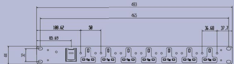
T-07H 7 WAY 1U HORIZONTAL
