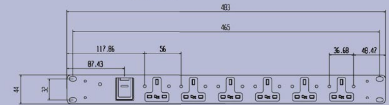
T-06H 6 WAY 1U HORIZONTAL
